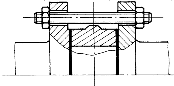
图 3 对夹连接
