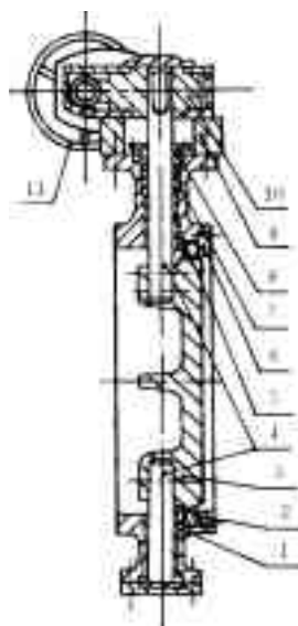
1—阀体; 2—阀体密封圈(阀座); 3—蝶板; 4—阀杆; 5—轴套; 6—压圈; 7—填料; 8—填料压盖; 9—连接座; 10—蜗轮减速箱; 11—手轮
