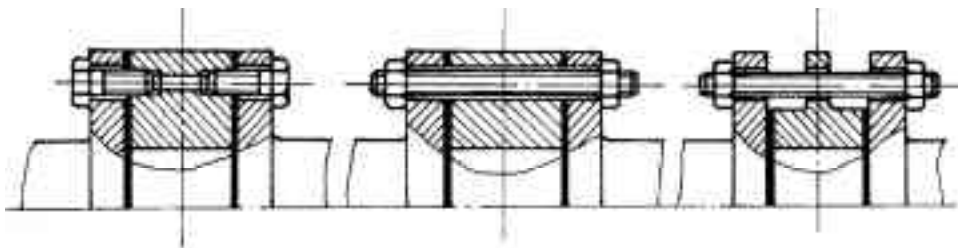
图 4 其他型式对夹连接
