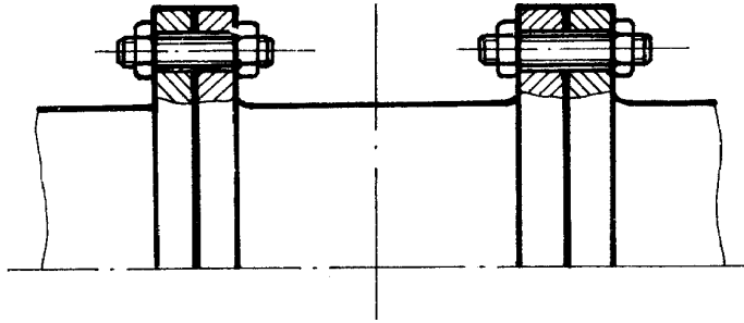
图 5 双法兰连接
