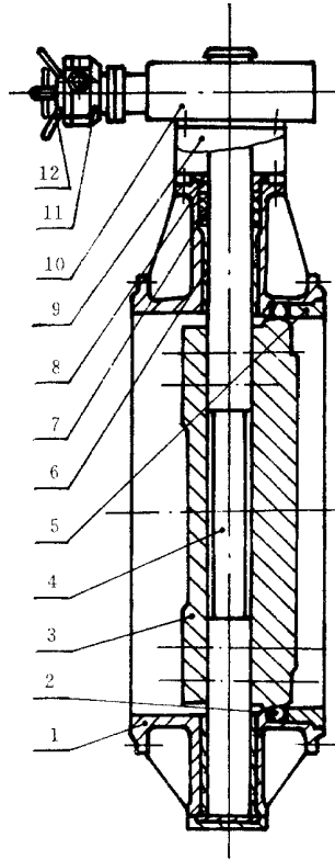
1—阀体；2—阀体密封圈(阀座)；3—蝶板；4—阀杆；5—压圈； 6—轴套；7—填料；8—填料压盖；9—隔热连接座；10—二级驱动装置；11—一级驱动装置；12—手轮 图 2 双法兰连接蝶阀
